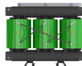
Tipo seco pequeno
