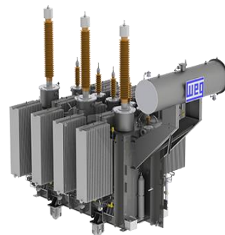
Transformador de grande potência (LPT)
